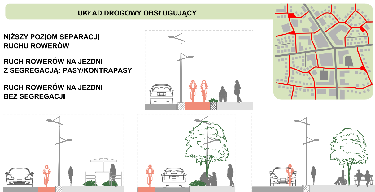
Rys. 10.2. Lokalizacja tras dla rowerów w ramach obsługującego układu drogowego
